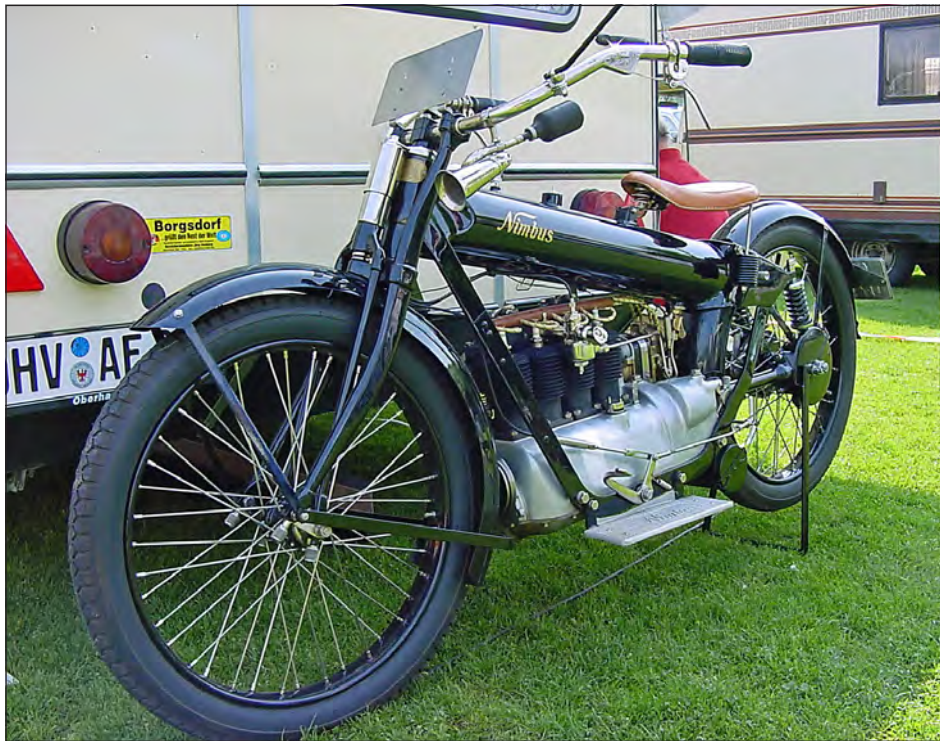
Die Nimbus A heißt wegen ihres markanten Tanks bei allen Motorradfreunden „Nimbus Offenrohr“. Fotos: Thomas Welzel
