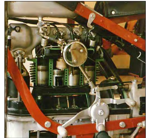
Im Schnittmodell sind die vier Zylinder des Reihensmotors sehr gut zu erkennen.
